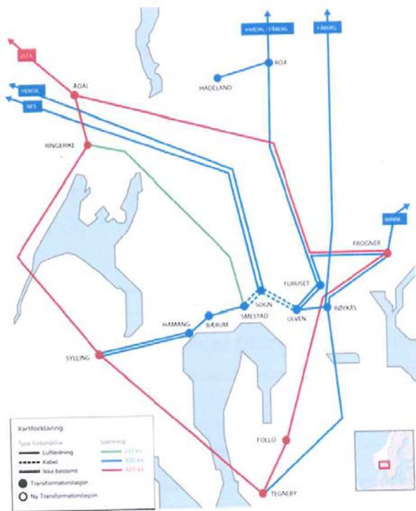
Figur 1: Dagens nettstruktur i Stor-Oslo (kilde: KVVU)
