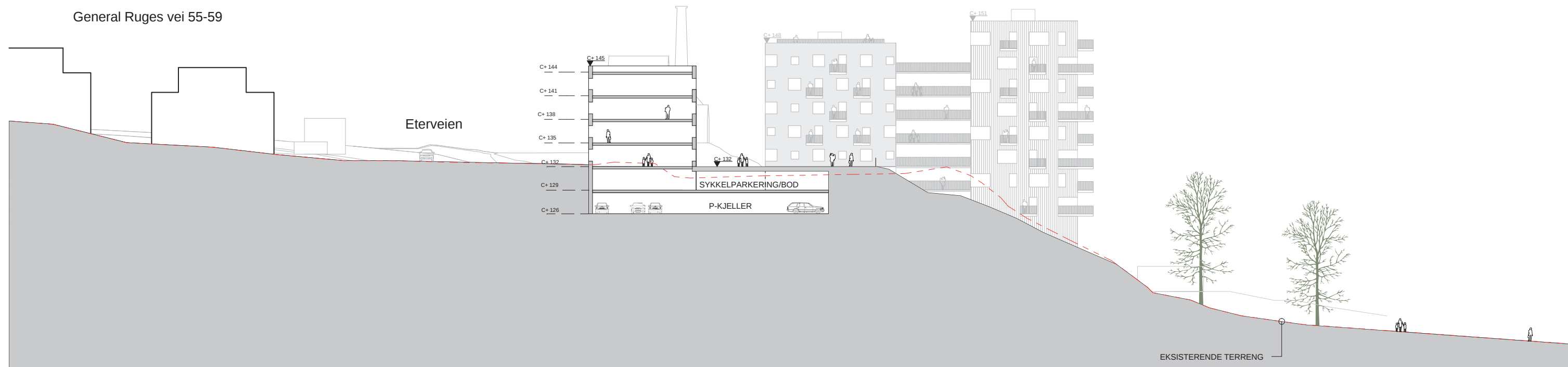
Tverrsnitt A-A'
