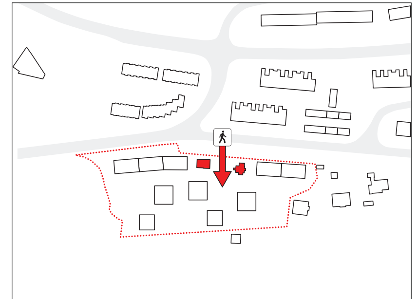
HOVEDADKOMST MELLOM EKSISTERENDE BYGG
