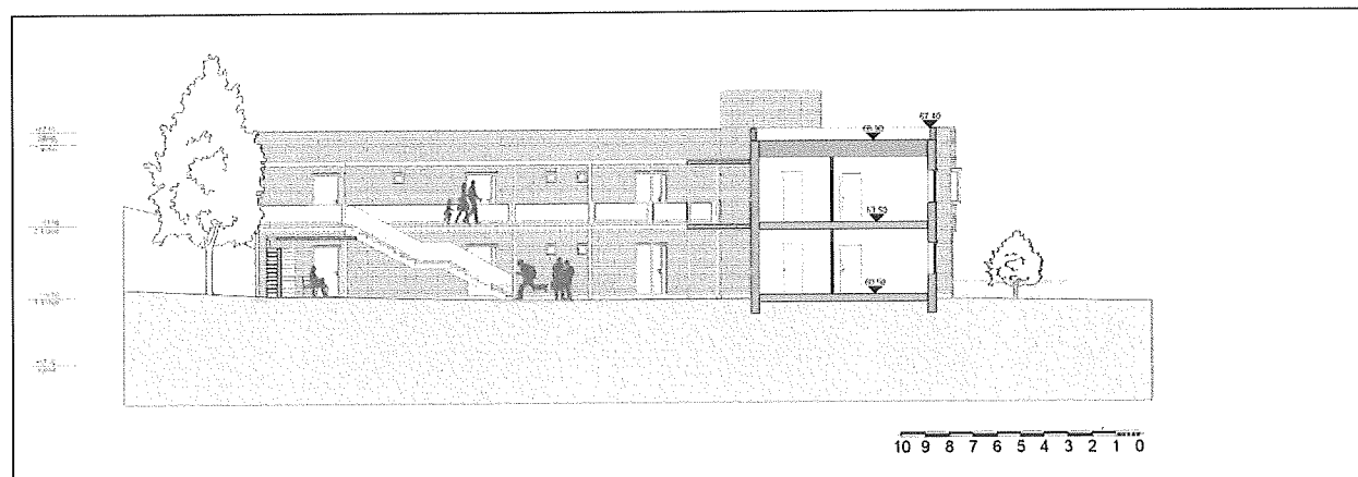
Snitt B-B
