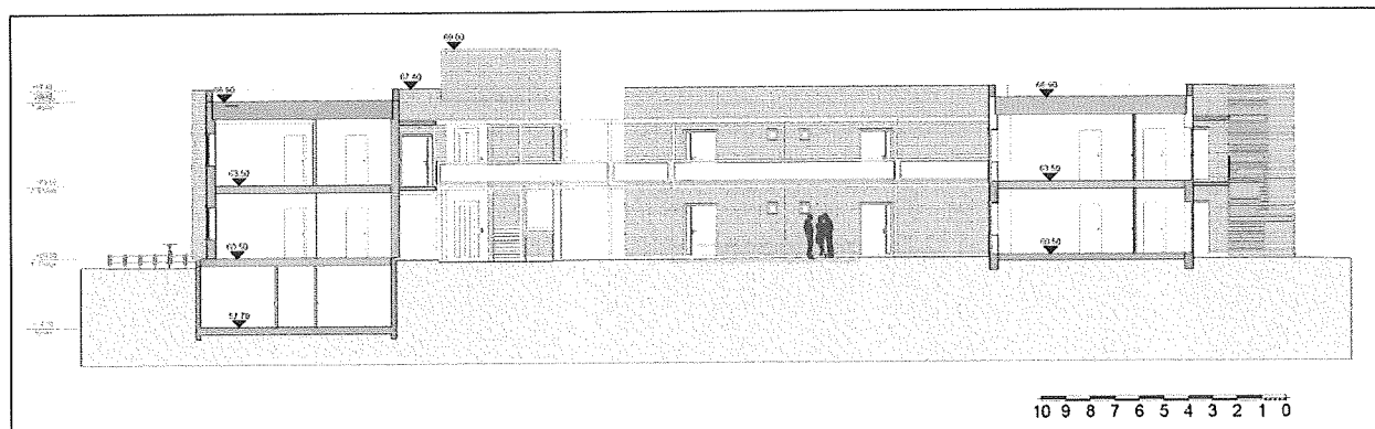
Snitt A-A
