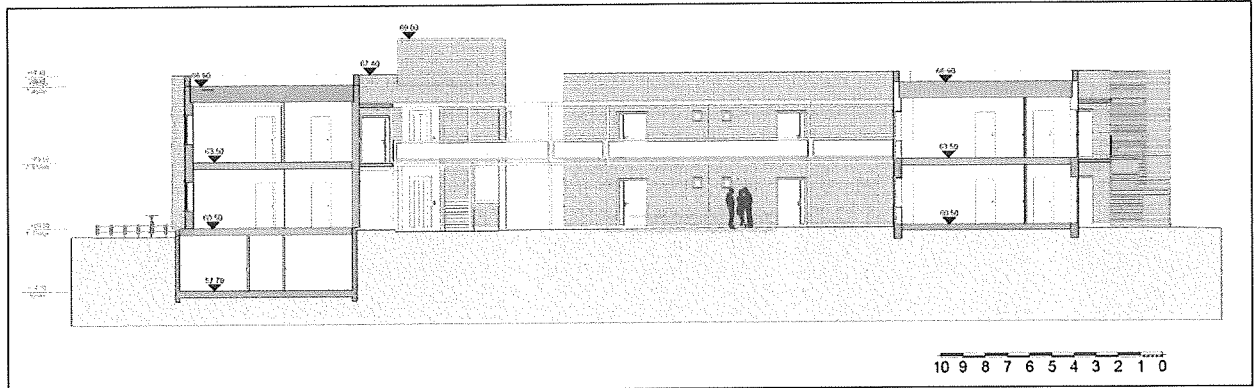
Snitt A-A
