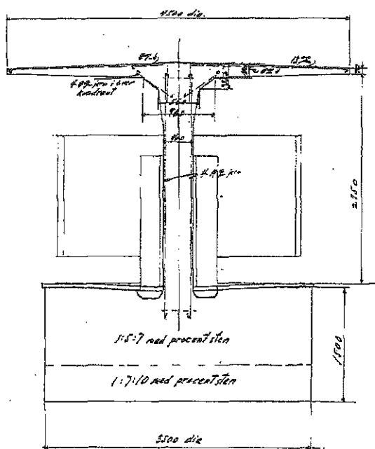
Snittegning av pissoaret slik det var planlagt i 1935.
