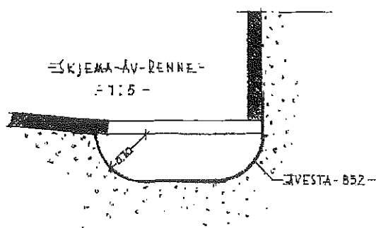
Snitt av renne 1937.
