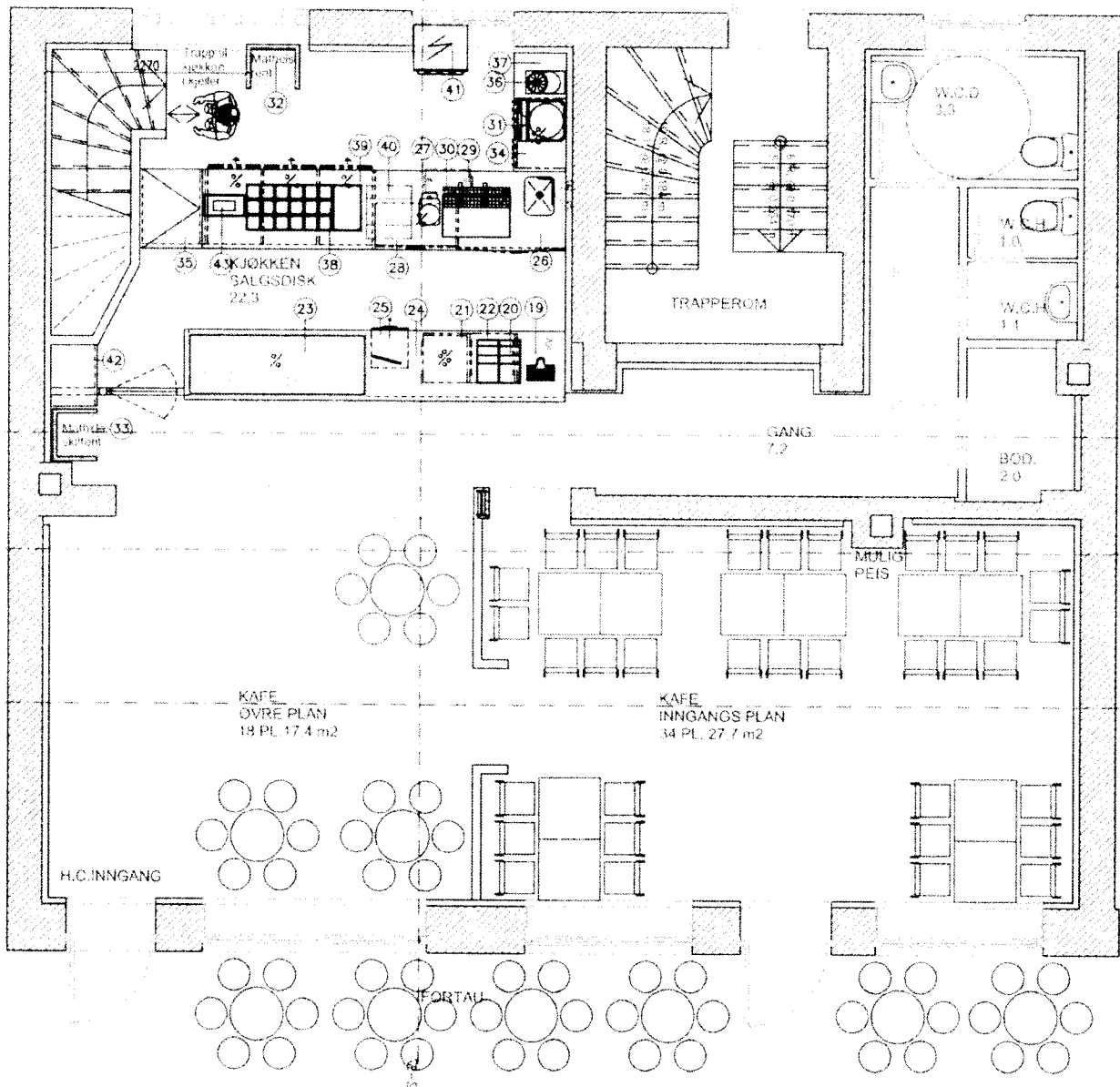
PLAN 1. ETASJE
