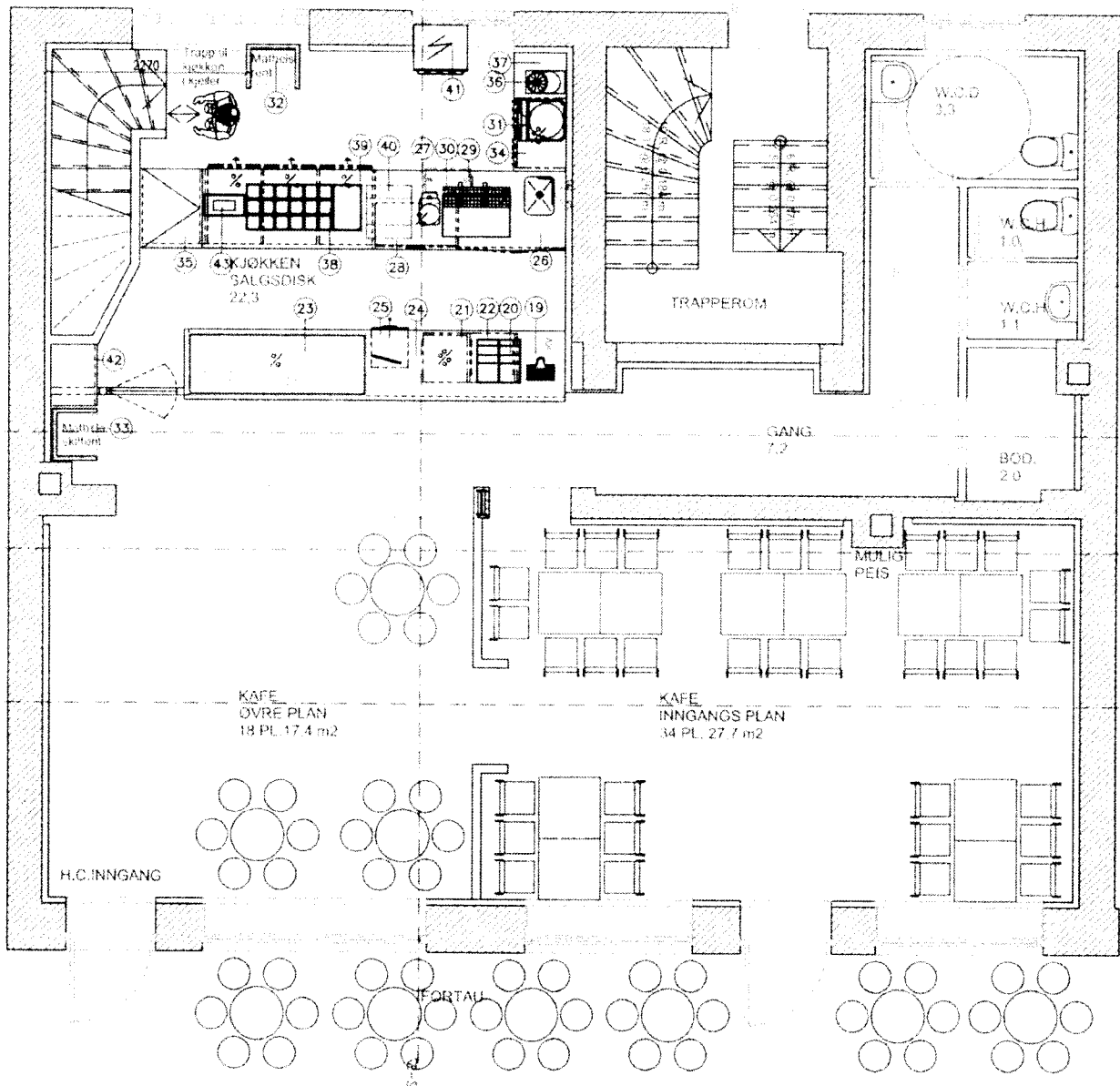
PLAN 1. ETASJE
